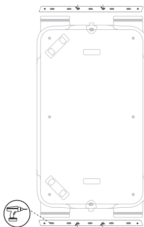
Instalace montážních konzolí – šířka jednotky
