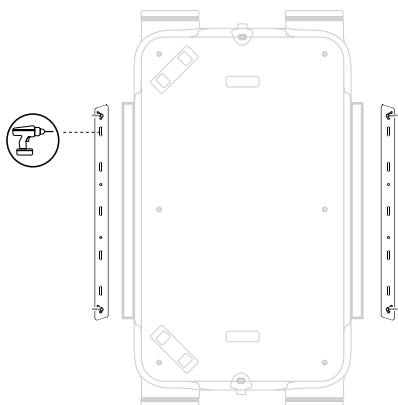
Instalace montážních konzolí – délka jednotky
