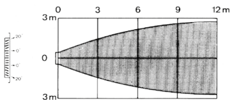
nastavení lamel 20°
