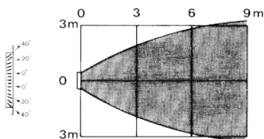
nastavení lamel 40°
