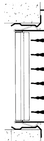
Mřížka s pružinami a montážním rámečkem
