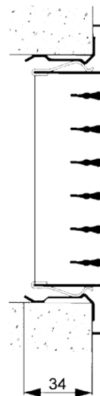
Mřížka s pružinami a montážním rámečkem
