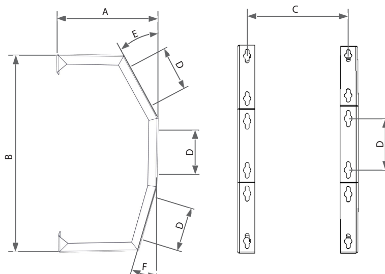
Rozměry konzolí
